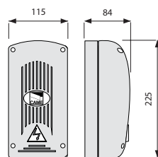
ZR24
